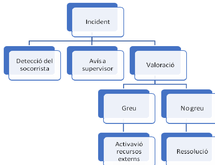
Fig.3 Resolució d'incidents
